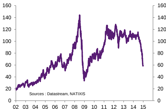
Graphique 11a Prix spot du pétrole (brent, $ par baril)
